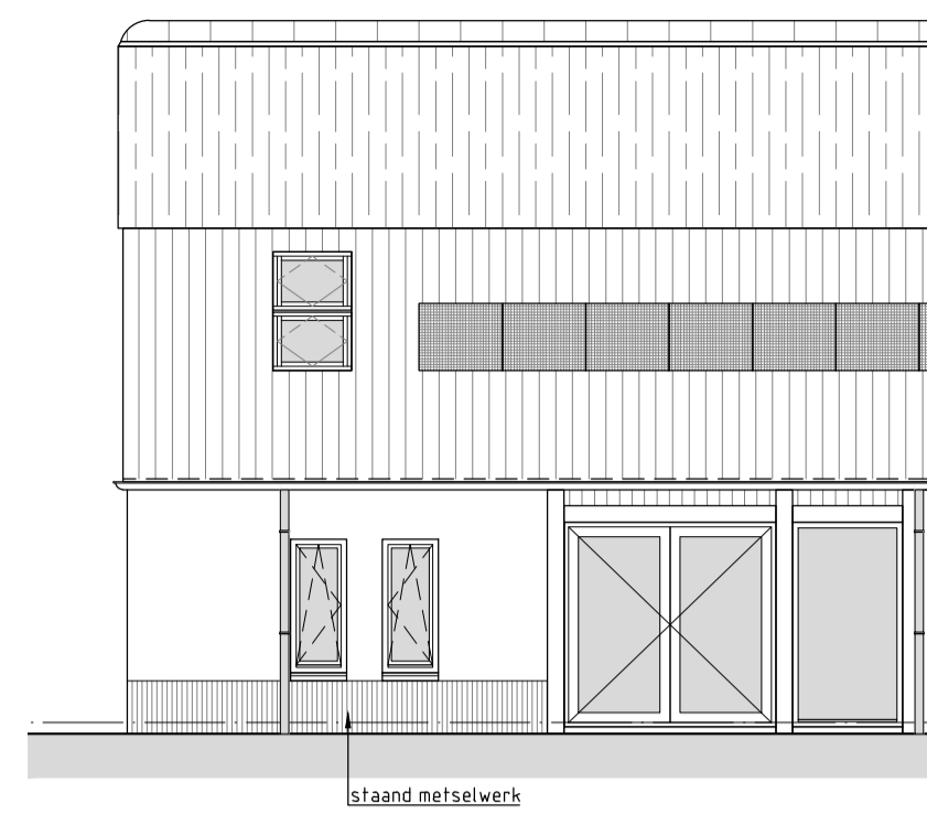
ACHTERGEVEL
