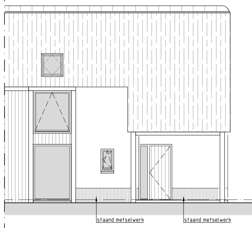
VOORGEVEL
