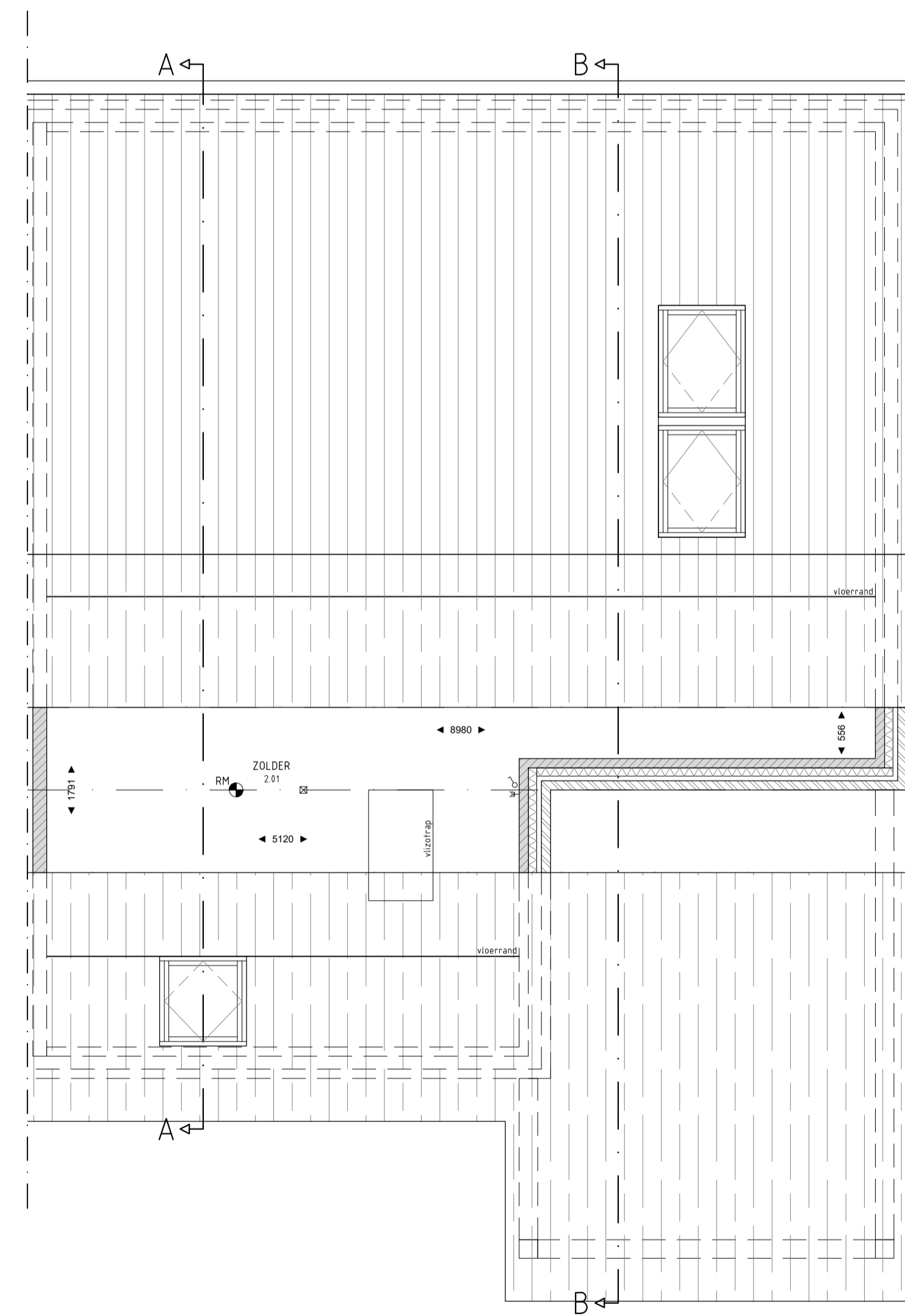
ZOLDER schaal 1:50
