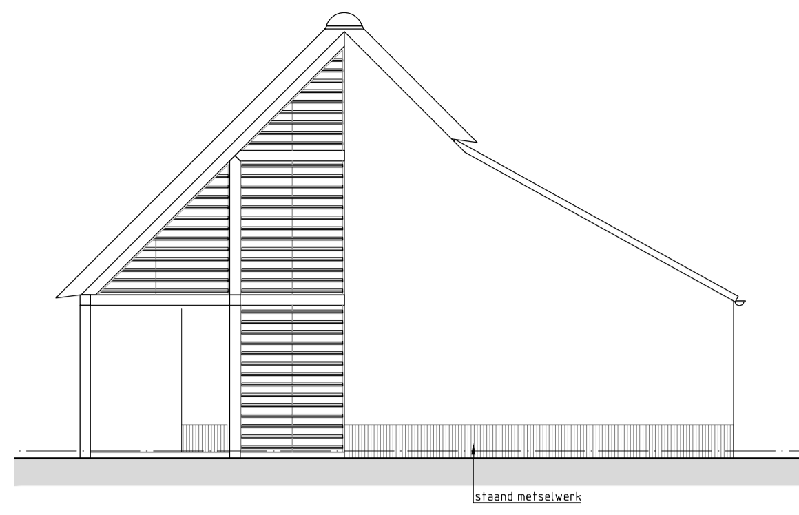
RECHTER ZIJGEVEL
