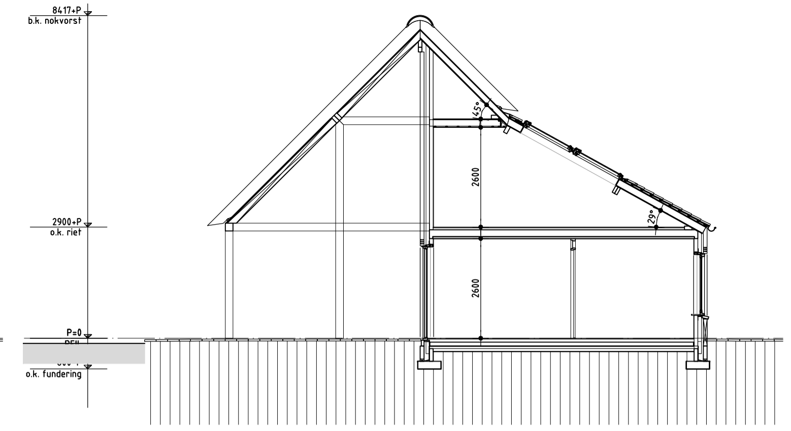
DOORSNEDE BB
